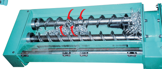
2軸スクリータイプ Double-shaft screw type
